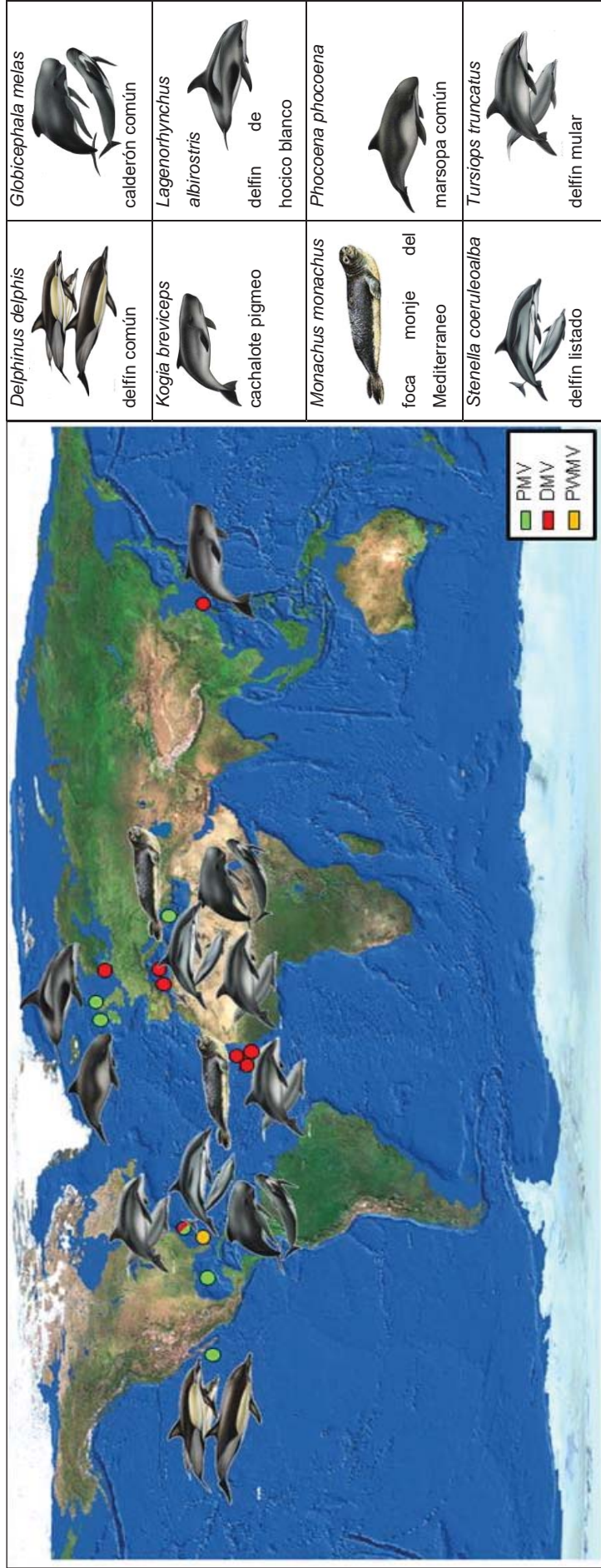
Figura 14. Situación geográfica de los diferentes tipos de CeMV detectados y caracterizados molecularmente
