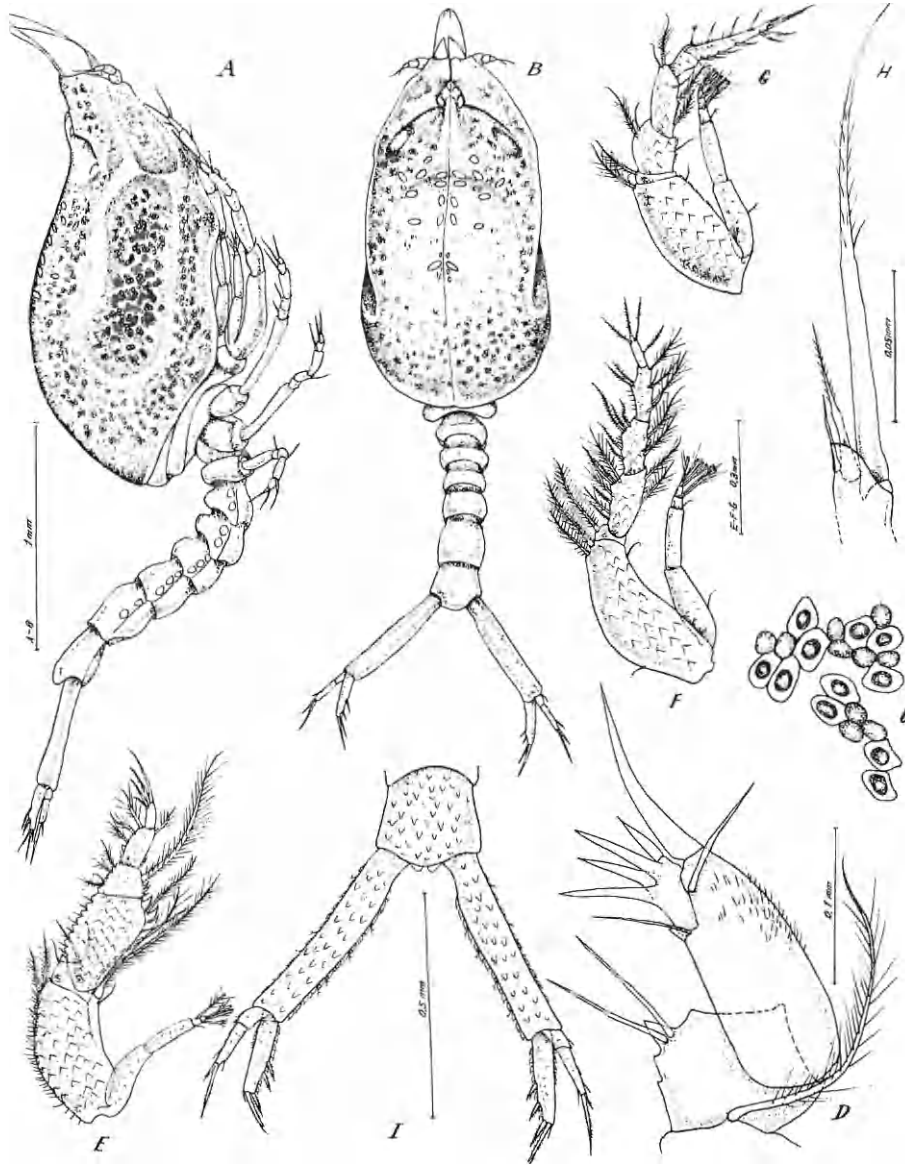
FIG. 5. — Campylaspis legendrei africana n. sp., femelle M. A. de profil ; B. vue d'en haut ; C. microstructure du tégument ; D. bout distal du maxillipède II ; E. maxillipède III ; F, G. péréiopodes I et II ; H. bout distal de son dactylopedite ; I. uropode (orig.).
