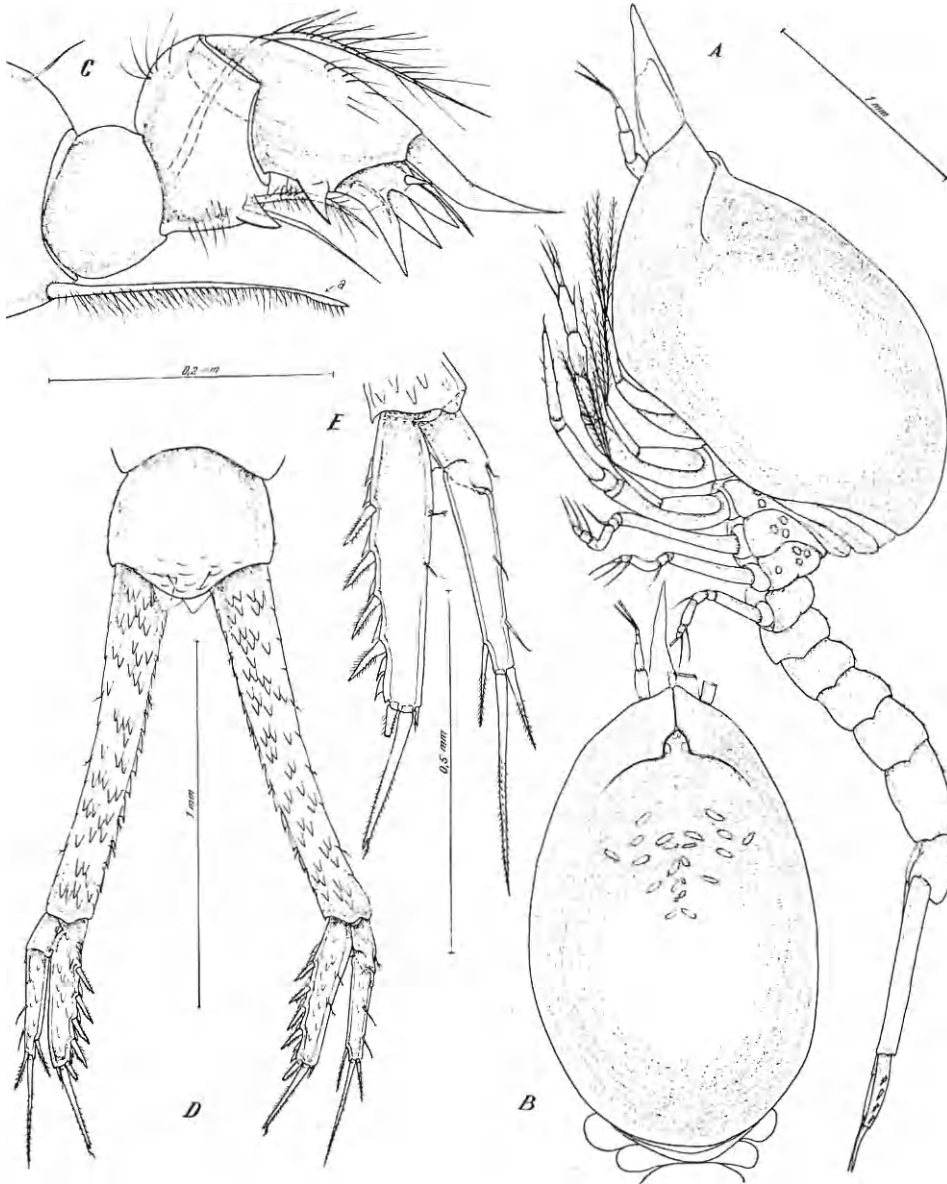
FIG. 2. — Campylaspis mauritanica n. sp., femelle P. A. de profil; B. vue dorsale de la carapace; C. portion distale du maxillipède II; a) bout gonflé du phallère séparé de son basipodite; D. uropode; E. branches des uropodes, agrandies (orig.).
