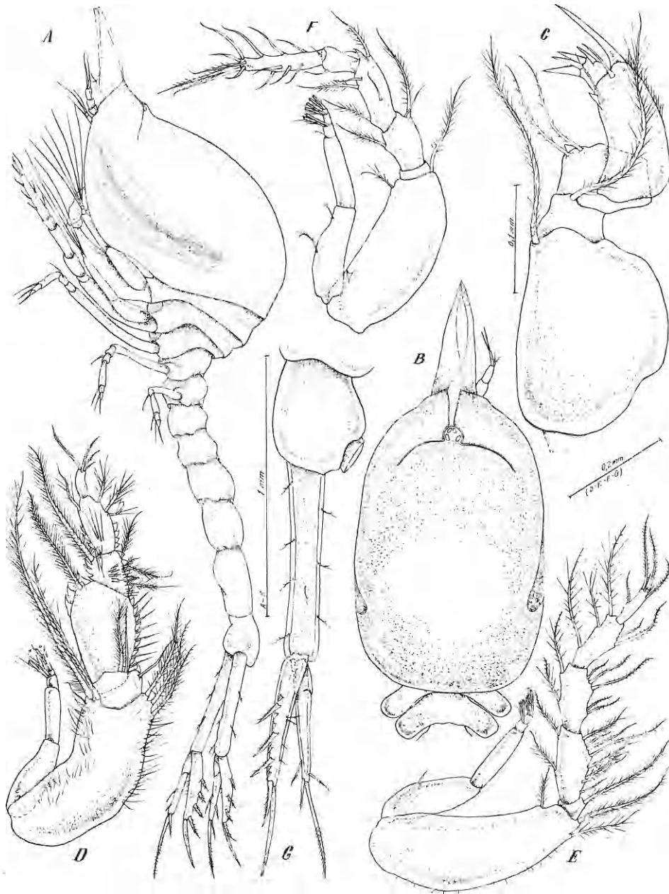
FIG. 6. — Campylaspis jonesi n. sp. B. mâle P, vue dorsale de la carapace; A à G, femelle juvénile, A. de profil; C. maxillipède II; D. maxillipède III; E. péréiopode I; F. péréiopode II; G. uropode (orig.).
