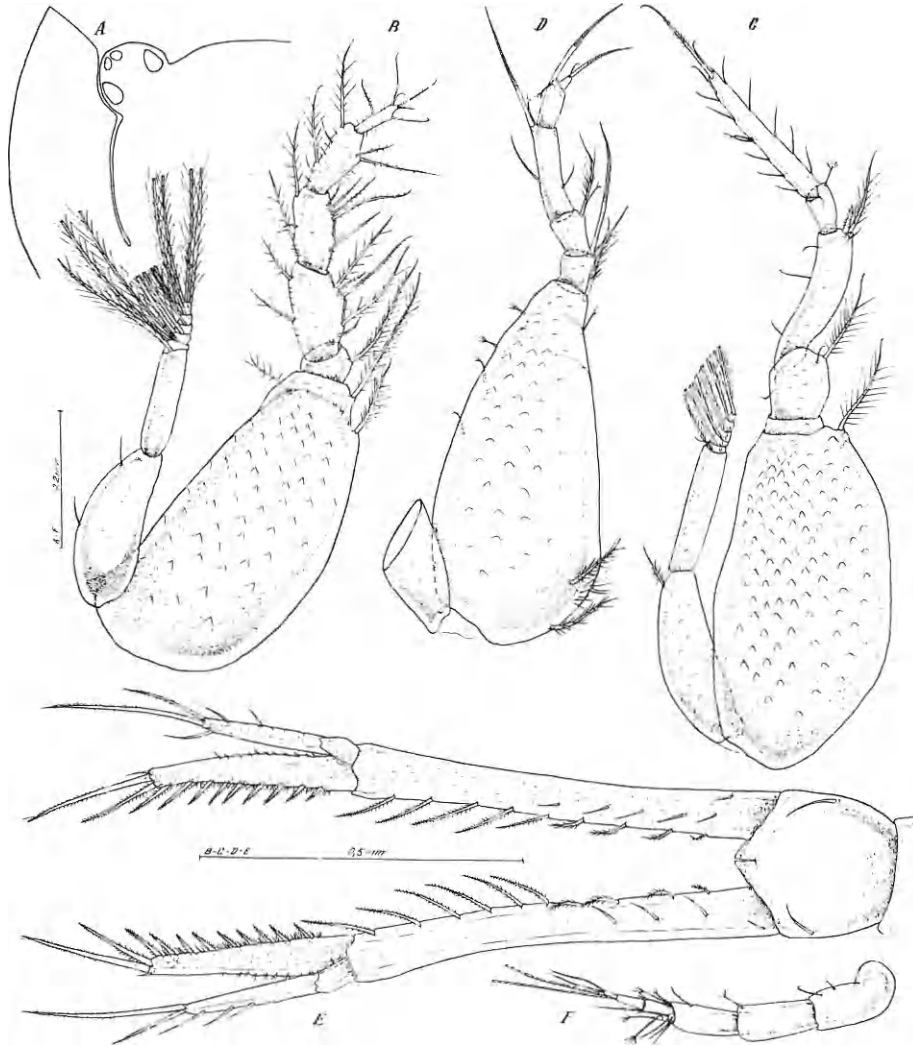
FIG. 4. — Campylaspis honetti n. sp., mâle adulte. A. lobes frontal, oculaire et pseudorostral, vue dorsale; B, C, D, respectivement péréiopodes I, II et III; E. uropode; F. antenne I. (orig.).
