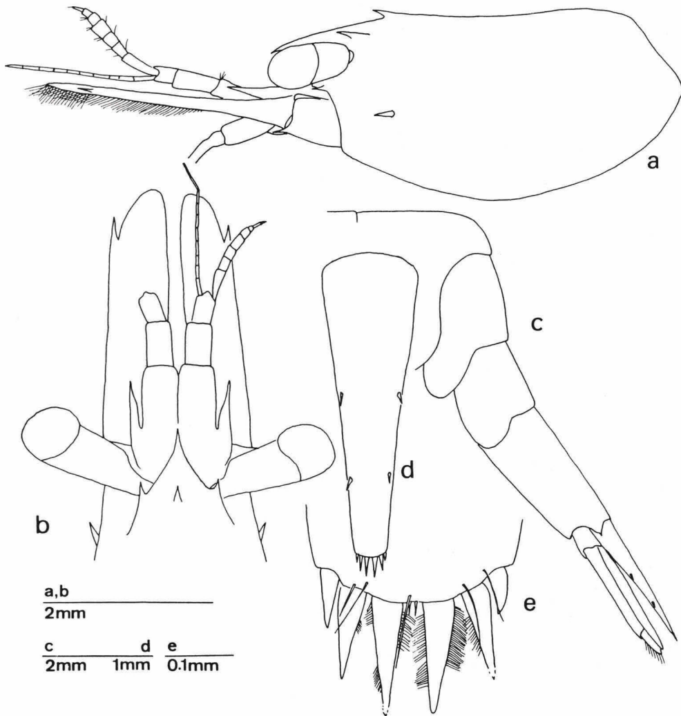
Fig. 40. Hippolyte sapphica d'Udekem d'Acoz forma B, NW Greece, Agia Triada [St. E8] (RMNH), mature females. a, cephalothorax; b, anterior part of cephalothorax in dorsal view; c, posterior part of pleon; d, telson; e, tip of telson.
