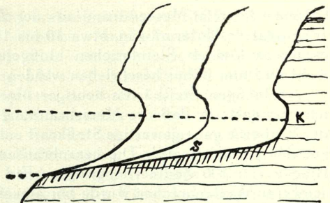
Abb. 2. Zurückweichen der felsigen Steilküste vor der Meeresbrandung. — Bildung von Schorre (S) und Kliff (K).
