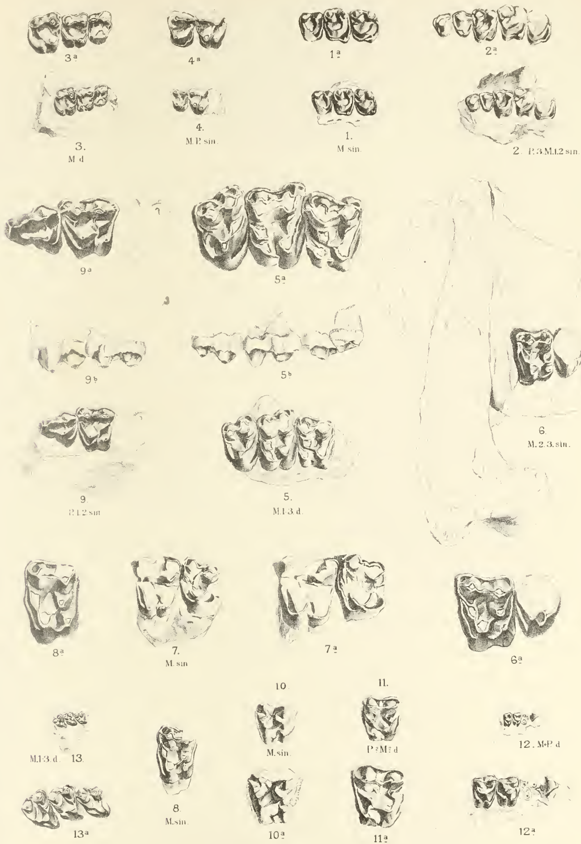
Fig. 1. 2. Caenopithecus lemuroides . Fig. 3. 4. Adapis Duvernoyi . Fig. 5-9. Phenacodus europaeus Fig. 10. Protofoënia . Fig. 11. Meniscodon . Fig. 12. Pelycodus ? Fig. 13. Mioclaenus ?
