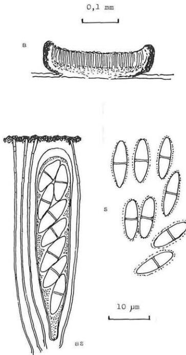
Abb. 1. Gyalidea culbersoniana spec. nova (Typus). – ap Vertikalschnitt durch ein Apothecium, as Ascus und Paraphysen, sp Ascosporen.
