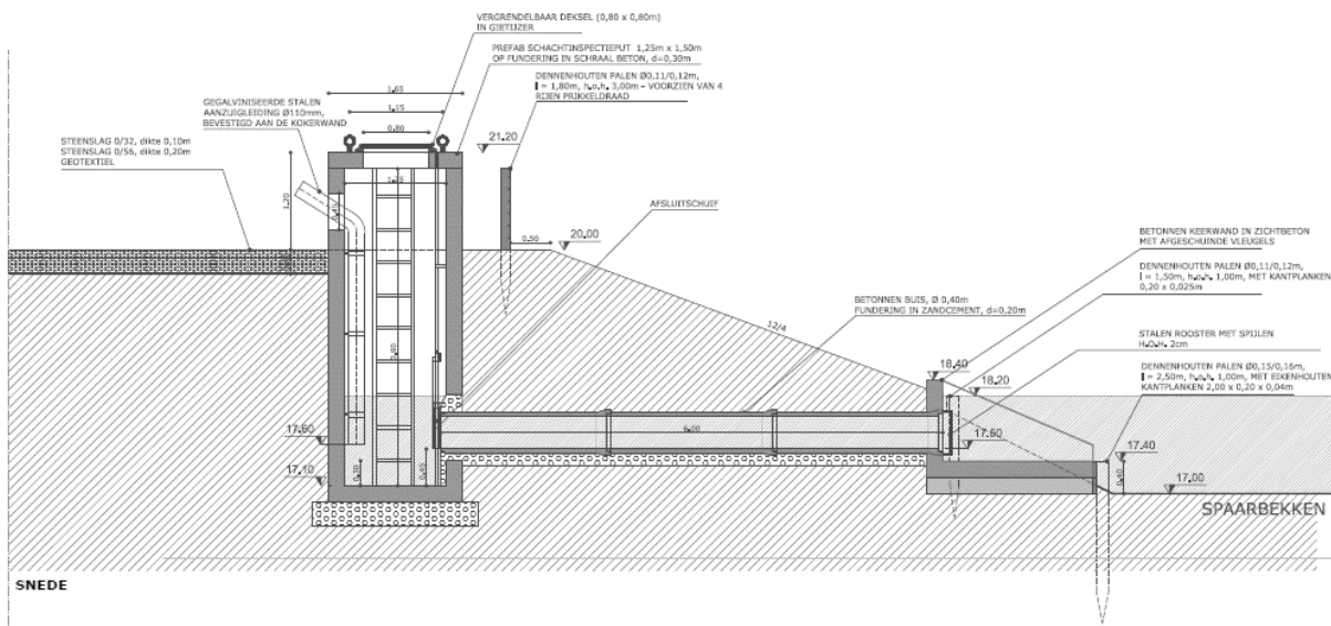
Figuur 7: principe dwarsdoorsnede captatiepunt
